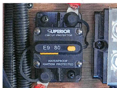
ブレーカー
